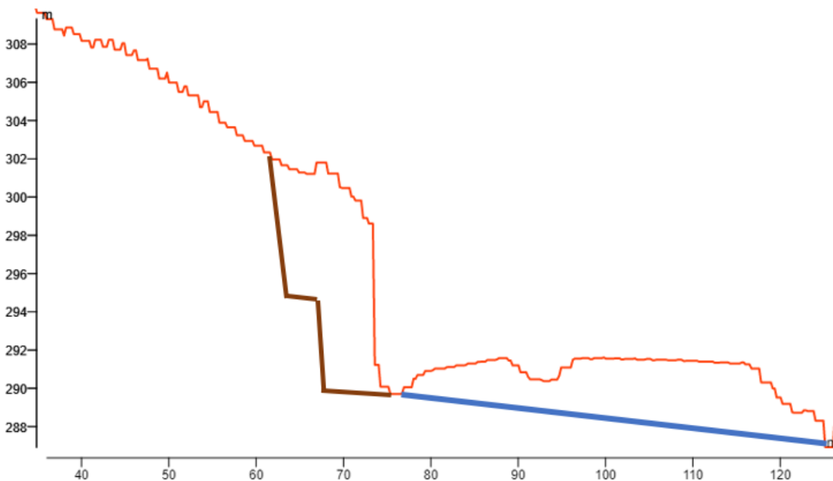
Figur 5-32. Eksempel på prinsipløsning for bekkekryssing ved profil 35180.
