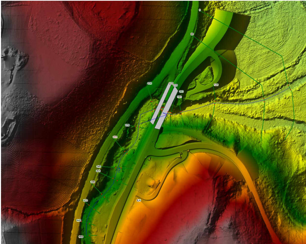
Figur 5-51. 1D HEC-RAS-modell av Fossemsbrua for planlagt situasjon. Grønne linjer er tverrprofiler. Blå linje er senterlinje elv basert på terrengmodell
