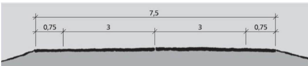
Figur 6: Tverrprofil H1, 7,5 meter og ÅDT 4000 – 12 000. (Kilde: Statens vegvesen Håndbok N100, 2014).
