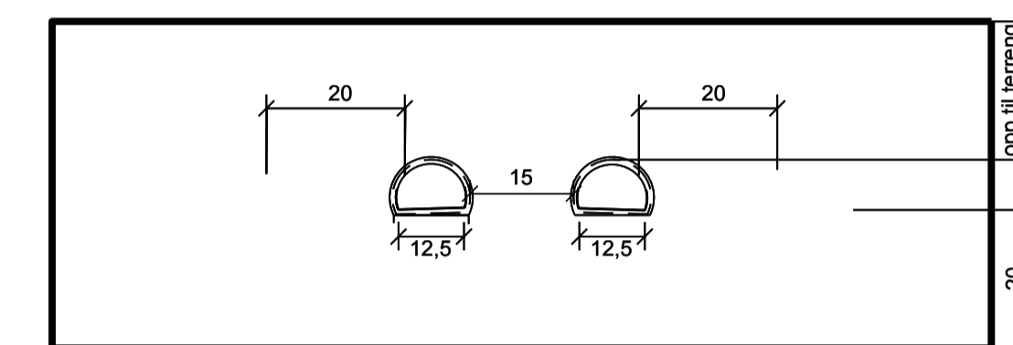
Vegttunnel med havarilomme med sikringszone
