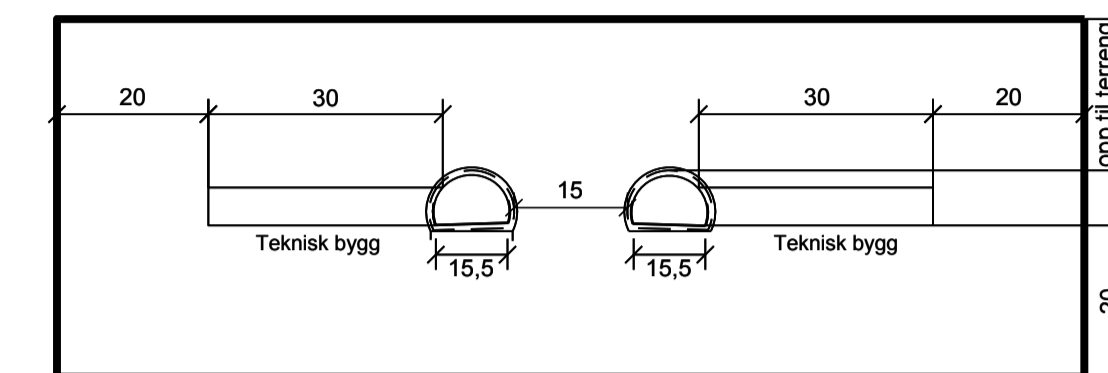
Vegttunnel med havarilomme og teknisk bygg med sikringszone
